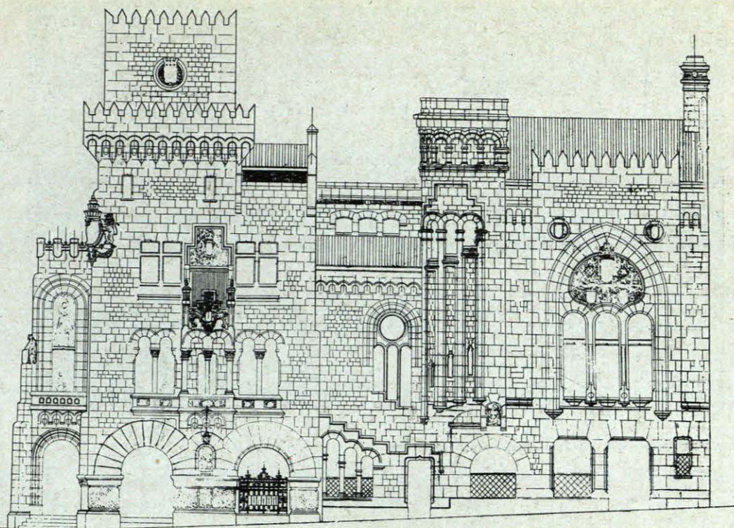
Alzado principal.
