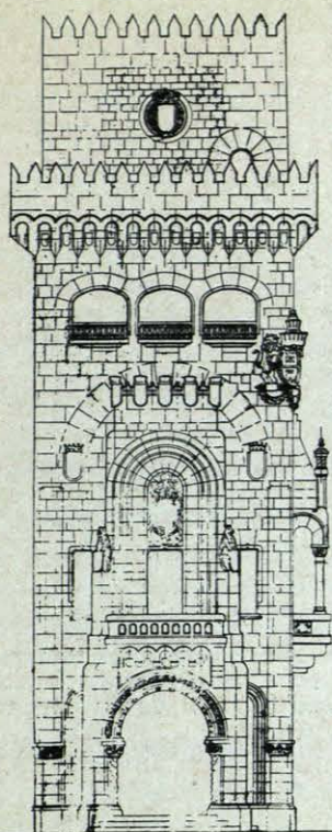
Alzado lateral.
